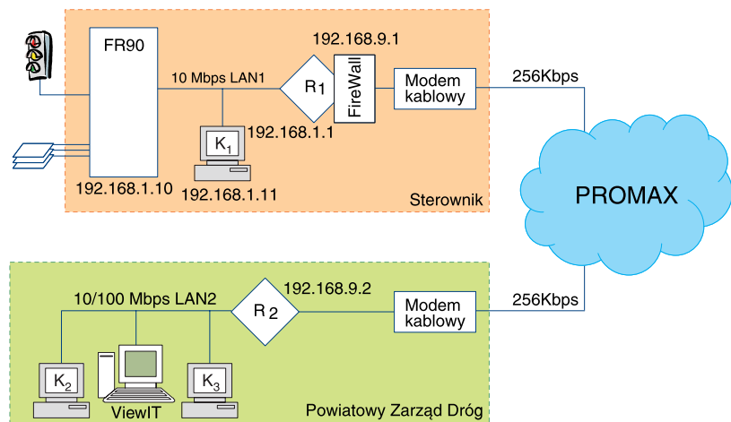
Rys. 2. Struktura sieci telematycznej
