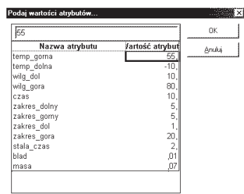
Rys. 1. Ekran programu PC Shell (wybór wartości atrybutów) Fig. 1. Screen of PC Shell program (choose value of attribute)
