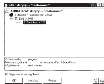
Rys. 2. Ostatni ekran programu PC Shell
