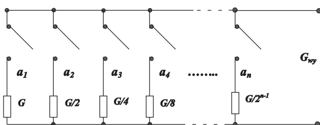
Rys. 3. Schemat dwójnikowego symulatora konduktancji
