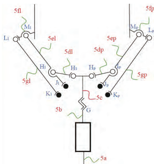
Rys. 3. Struktura kinematyczna chwytaka robota SCOUT
