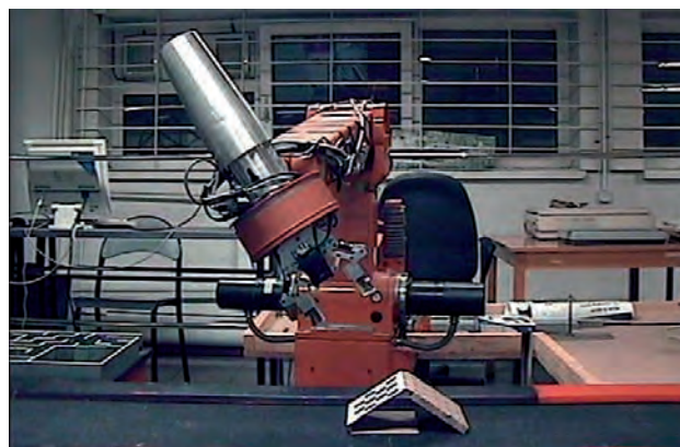
Rys. 10. Manipulator IRp-6 nad szachownicą podczas serwowizji Fig. 10. The IRp-6 manipulator above the chessboard during visual servoing
