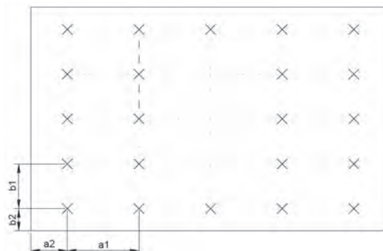
Rys. 1. Przykład rozmieszczenia opraw oświetleniowych Fig. 1. Example of luminaires layout spacing
