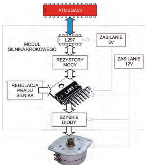
Rys. 6. Układ sterowania silnikiem krokowym Fig. 6. Stepper motor control system
