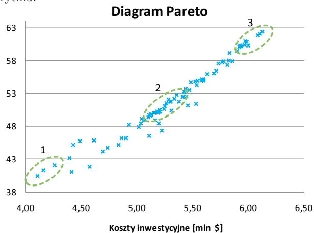
Rys. 3. Linia Pareto dla optymalizacji Sprawność egzergetyczna – koszty
