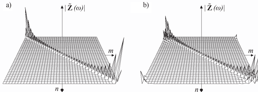
Rys. 2. Widmowe operatory impedancji (część rzeczywista) dwójników: a) stacjonarnego SLS, b) niestacjonarnego SLN
