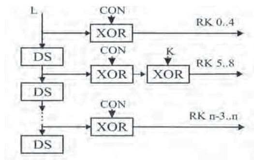
Rys. 4. Moduł Key Expand
