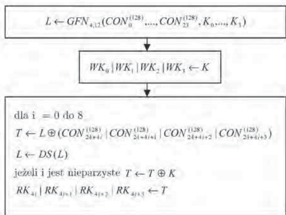
Rys. 2. Generacja podkluczy dla klucza 128-bitowego
