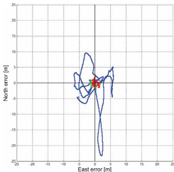
Rys. 7. Wykres wyznaczonych pozycji dla 3 odbiorników pracujących z różnymi systemami GNSS dla scenariusza I
