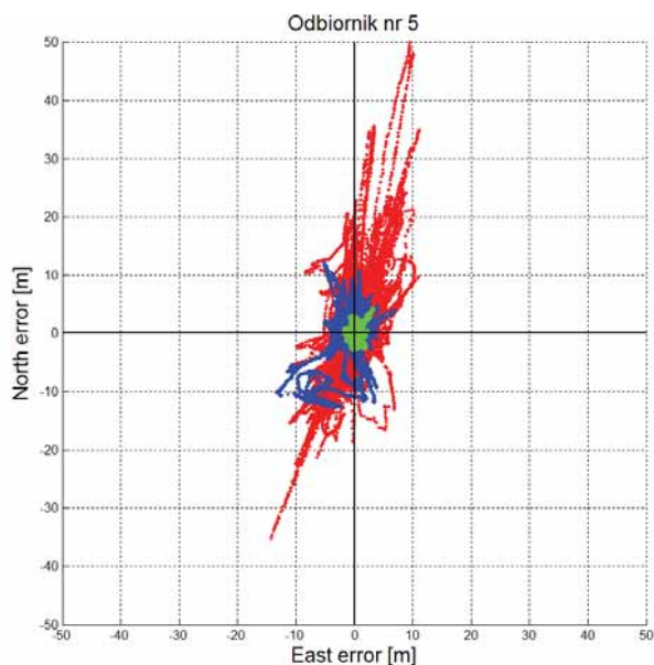
Rys. 6. Wspólny wykres dla wyznaczonych pozycji odbiornika starszej generacji dla 3 scenariuszy pomiarowych
