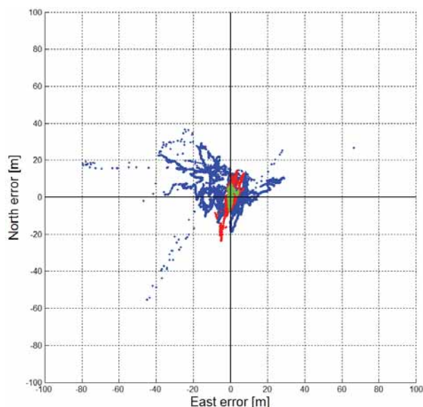
Rys. 8. Wykres wyznaczonych pozycji dla 3 odbiorników pracujących z różnymi systemami GNSS dla scenariusza III
