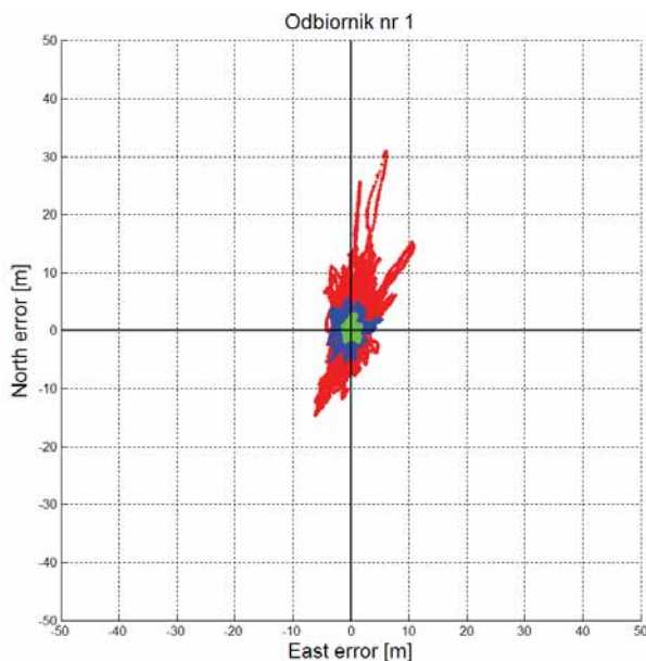
Rys. 5. Wspólny wykres dla wyznaczonych pozycji odbiornika nowszej generacji dla 3 scenariuszy pomiarowych
