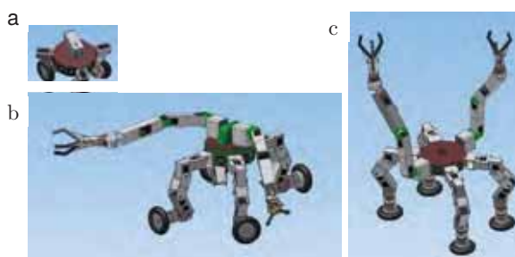
Rys. 10. Przykładowe konfiguracje robota Cameleon: a – robot trzykołowy z modułem wizyjnym, b – robot z czterema nogami zakończonymi kołami, wieżą i dwoma manipulatorami, c – robot czteroński z dwoma manipulatorami
