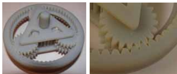
Rys. 2. Przekładnia planetarna wykonana z materiału VeroGray, z zastosowaniem technologii PolyJet
