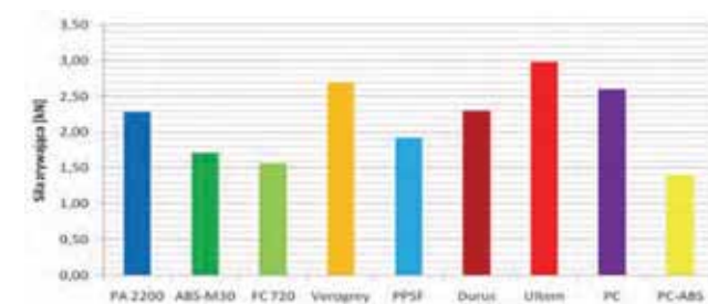
Rys. 5. Zestawienie wyników próby na rozciąganie
