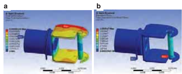
Rys. 13. Wyniki analizy wytrzymałościowej przykładowej części robota
