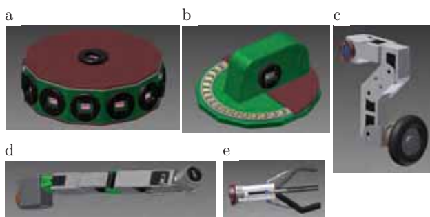
Rys. 9. Modele CAD wybranych modułów robota: a – korpus, b – wieża, c – pedipulator z modułem hybrydowym koło-stopą, d – manipulator, e – chwytak
