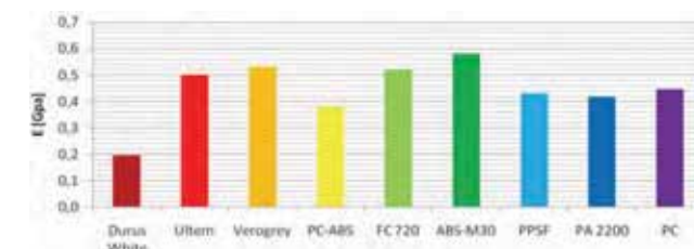
Rys. 7. Zestawienie wyników testu na wyznaczenie modułu Young'a na podstawie zginania dwupodporowego
