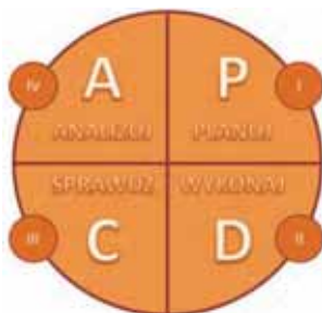
Rys. 2. Cykl Shewharta [4]
