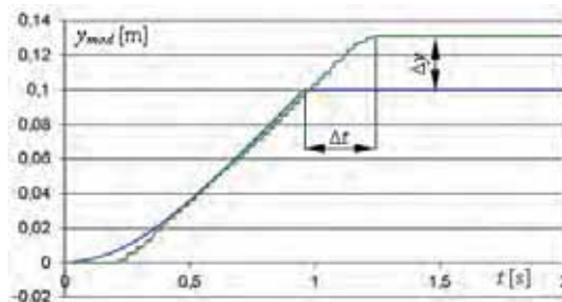
Rys. 8. Przebiegi położenia dżojstika i siłownika w układzie bez sprzężenia dotykowego
