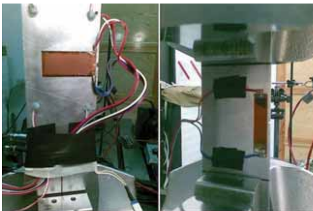
Fig. 5. Flat specimen view, front and back side Rys. 5. Widok płaskiej próbki, strona przednia i tylna
