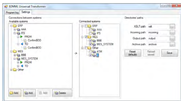
Rys. 4. Zakładka Settings
