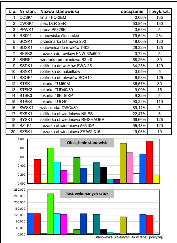
Rys. 6. Przykładowe wyniki z symulacji Fig. 6. Examples of results from simulation
