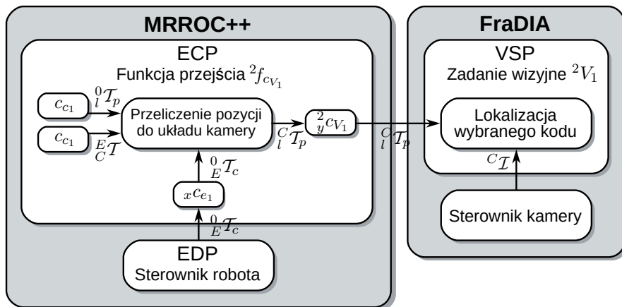
Rys. 7. Diagram przepływu danych funkcji przejścia {}^2f_{c_{V_1}}
