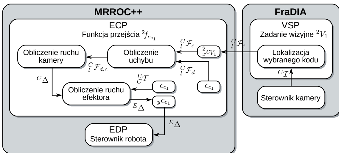
Rys. 8. Diagram przepływu danych funkcji przejścia {}^2f_{c_{e_1}}
