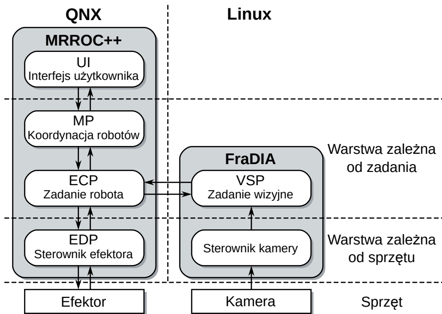
Rys. 2. Struktura sterowników ze sprzężeniem wizyjnym opartych na MRROC++ i FraDIA
