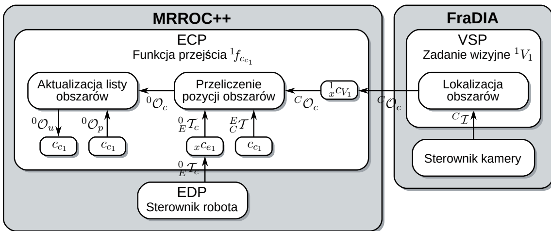
Rys. 6. Diagram przepływu danych funkcji przejścia {}^1f_{ce1}
