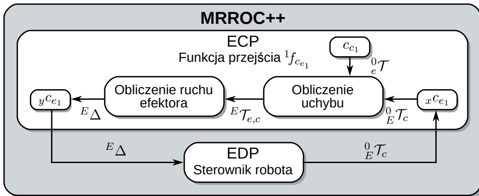
Rys. 5. Diagram przepływu danych funkcji przejścia {}^1f_{ce1}
