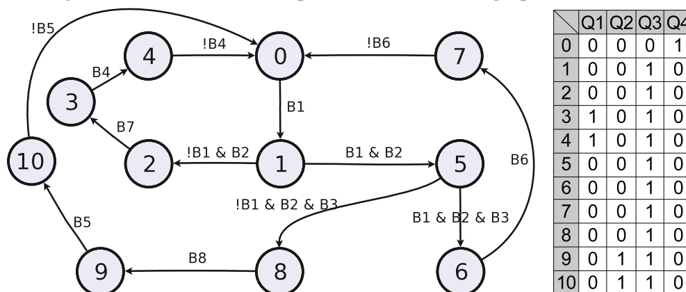
Rys. 5. Automat Moore'a i tablica wyjść stanów sortowniczy
