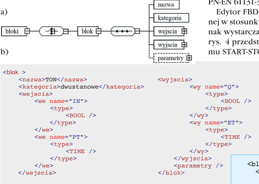
Rys. 2. a) Struktura biblioteki bloków edytora FBD; b) reprezentacja bloku TON w bibliotece
