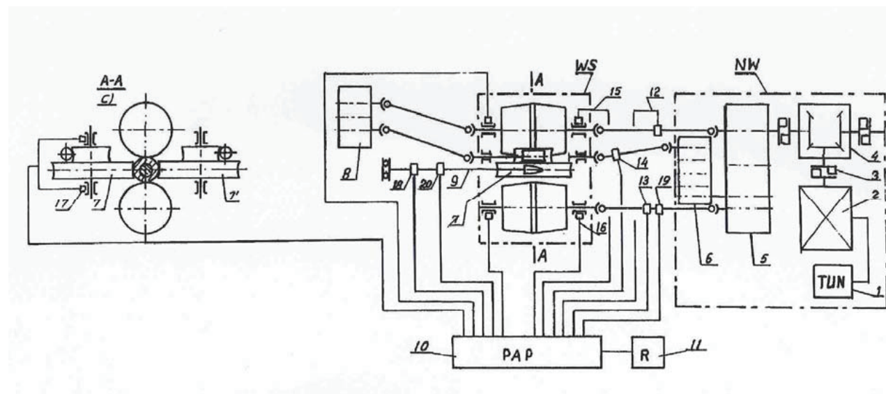
Rys. 5. Schemat laboratoryjnej walcarki skośnej [9]
