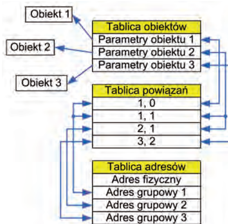
Rys. 2. Tablice konfiguracyjne urządzenia KNX
