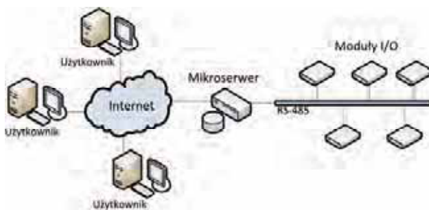
Rys. 1. Architektura systemu
