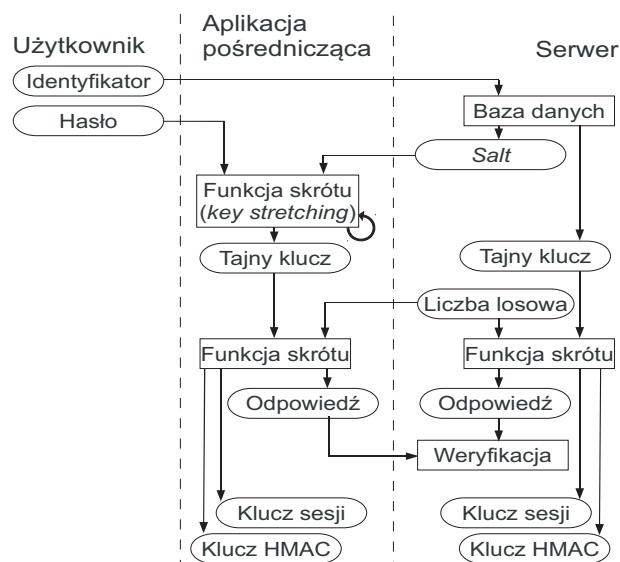
Rys. 2. Implementacja protokołu challenge-response
