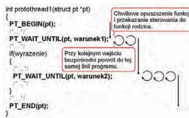
Rys. 5. Właściwości protothreadów
