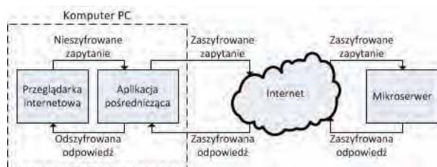
Rys. 6. Przepływ danych pomiędzy klientem i serwerem
