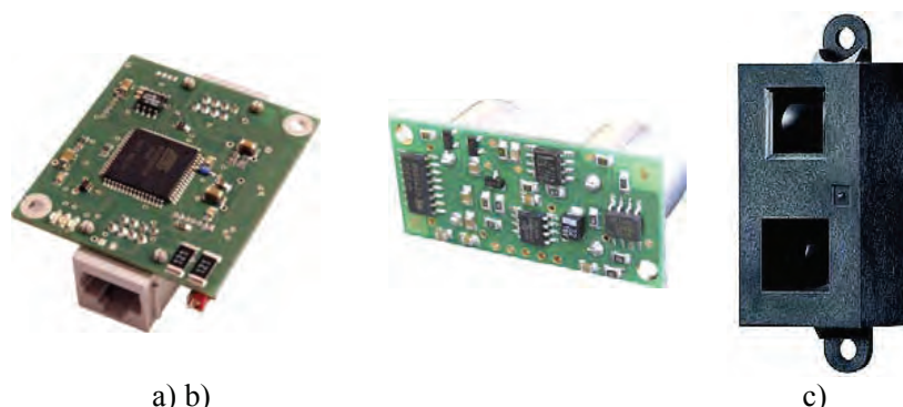
Rys. 12. Elementy sieciowego systemu sensorycznego, a) moduł sensoryczny, b) sensor US, c) sensor IR
