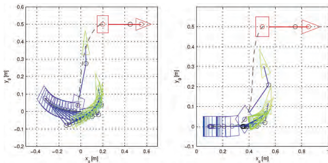
Rys. 9. Wyniki realizacji zadania śledzenia trajektorii (lewy: ruch tyłem) oraz sterowania do punktu (prawy: ruch przodem) w układzie sterowania VFO dla robota z przyczepą mocowaną pozaosiowo
