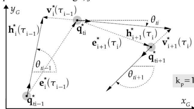
Rys. 4. Strategia planowania ruchu przez zbiór punktów przejazdowych
