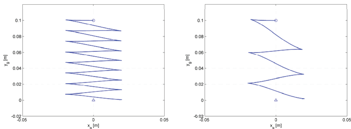
Rys. 10. Ścieżka pozycji dla robota dwukołowego w zadaniu parkowania z wykorzystaniem funkcji transwersalnych. Tunel błędny pozycji założono równy 0,02 m, dopuszczalny błąd orientacji 0,2 rad (po lewej) lub 0,5 rad (po prawej).
