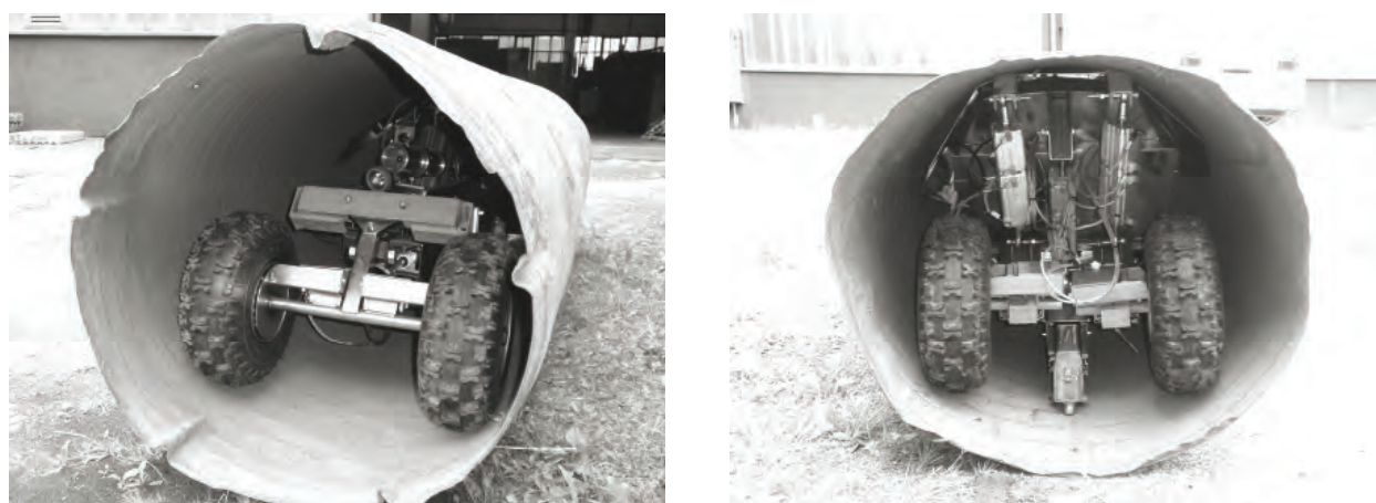
Rys. 9. Transport robota przez lutnię o średnicy 800 mm
