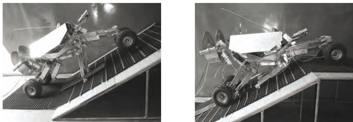
Rys. 7. Fazy wjazdu na wzdłużną rampę o nachyleniu 30°
