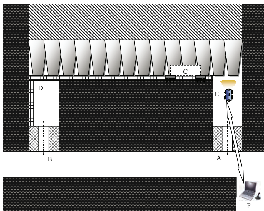
Rys. 1. Schemat poglądowy otamowanego rejonu ściany monitorowanej robotem A/B – przeciwwybuchowa tama wlotowa/wylotowa z przepustem tamowym o średnicy 80 cm, C – kombajn, D – przenośniki, E – robot inspekcyjny, F – konsola operatora
