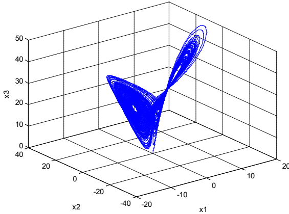
Rys. 1. Atraktor Lorenza
