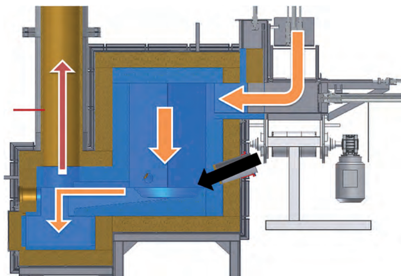
Rys. 3. Przekrój poprzeczny reaktora plazmowego z uwidocznionym kierunkiem przepływu odpadów i wytopu (pomarańczowe strzałki z góry do dołu), spalin (czerwona strzałka), oraz plazmy (czarna strzałka)
